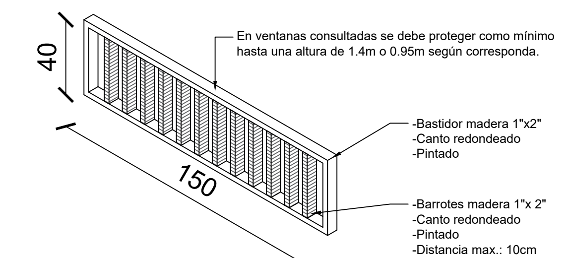
DETALLE INTERVENCIONES DETALLE DE VENTANAS ESCALA 1/25
