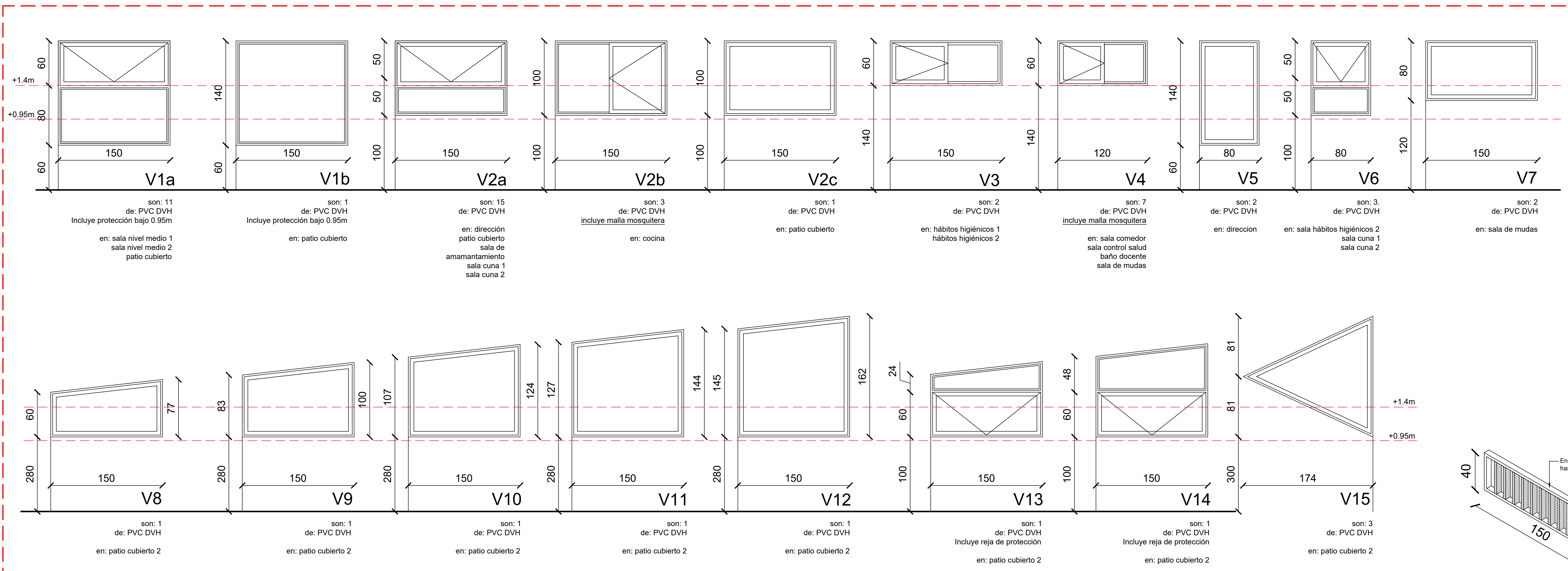
DETALLE INTERVENCIONES VENTANAS ESCALA 1/25
