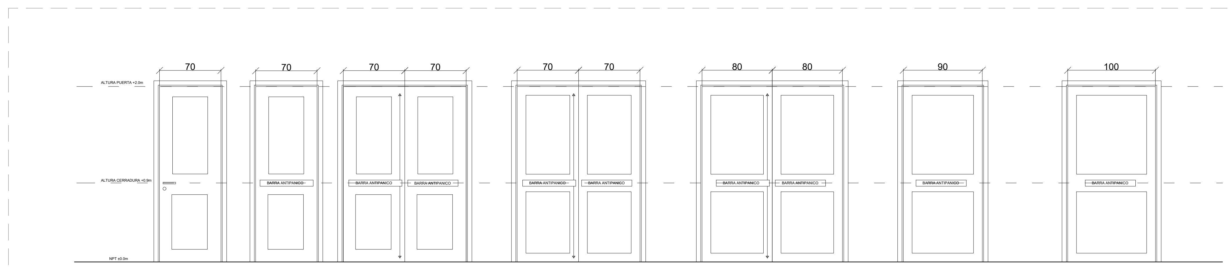
DETALLES DE PUERTAS ESCALA 1/25
